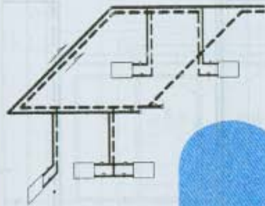
双管上供上回同程式
