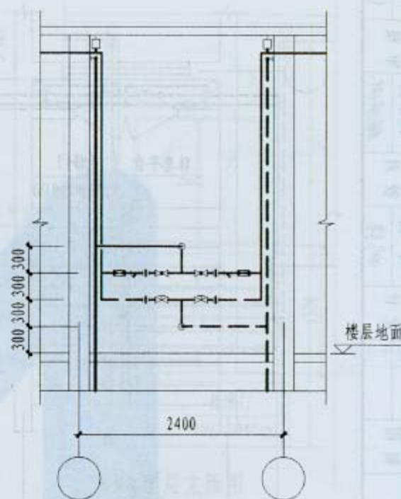
顶层立面图
