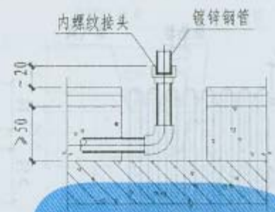
A-A剖面图
