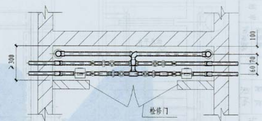
管道井平面图
