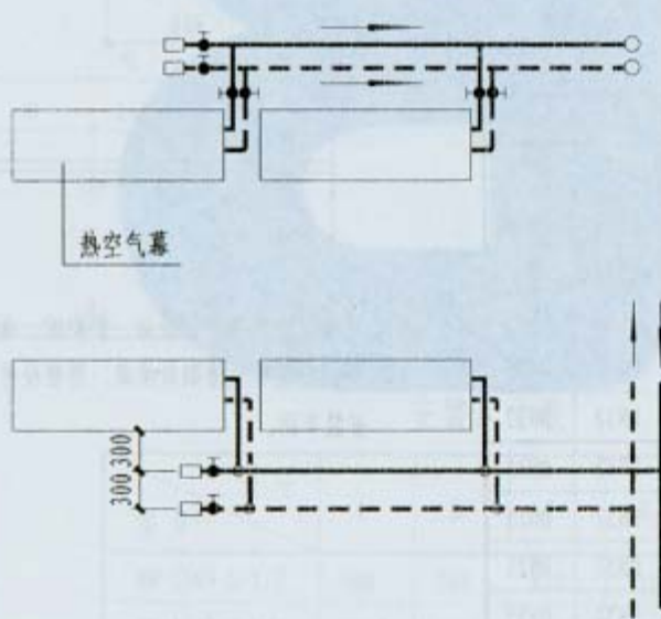
热水热空气幕配管图
