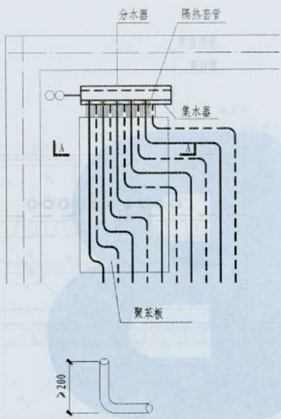
隔热套管
