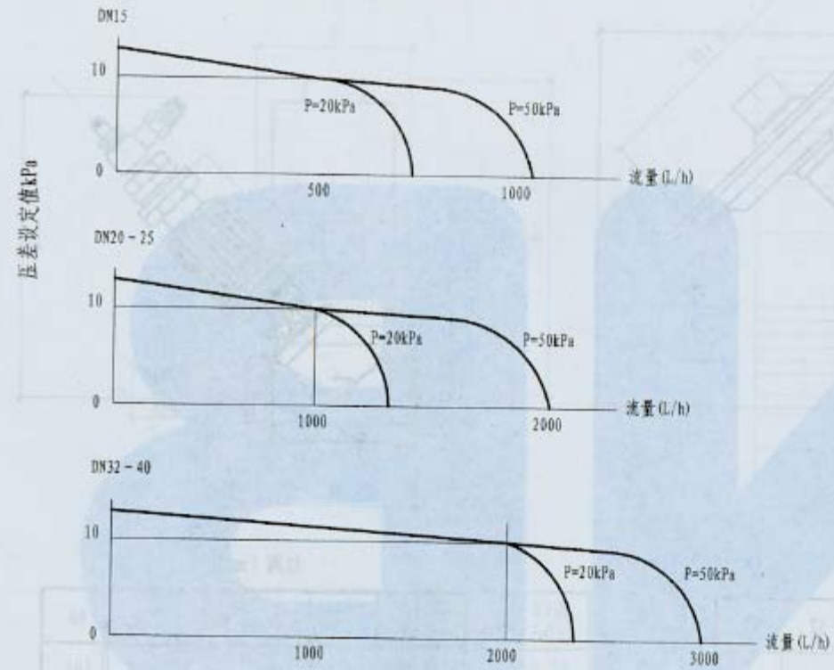
外网压差为20~50kPa流量特性曲线
