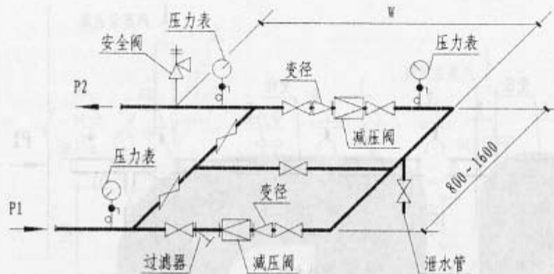
减压阀并排安装示意图
