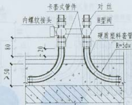
A-A剖面图
