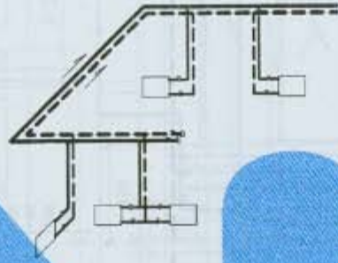
双管上供上回异程式
