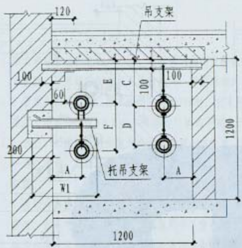
F 型
