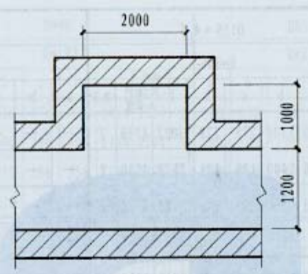
1 号井
