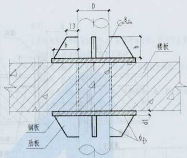
A-A 剖面
