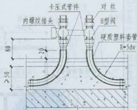
A-A剖面图
