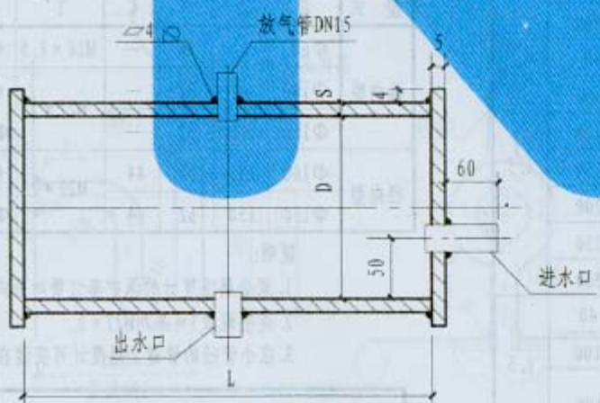
卧式集气罐
