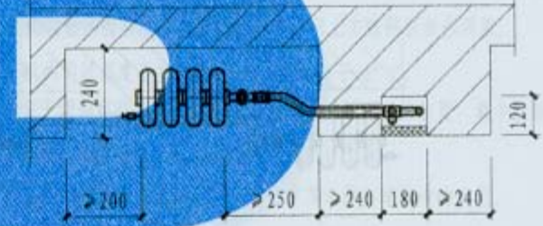
暗管散热器暗装平面
