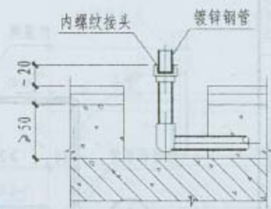
B-B剖面图
