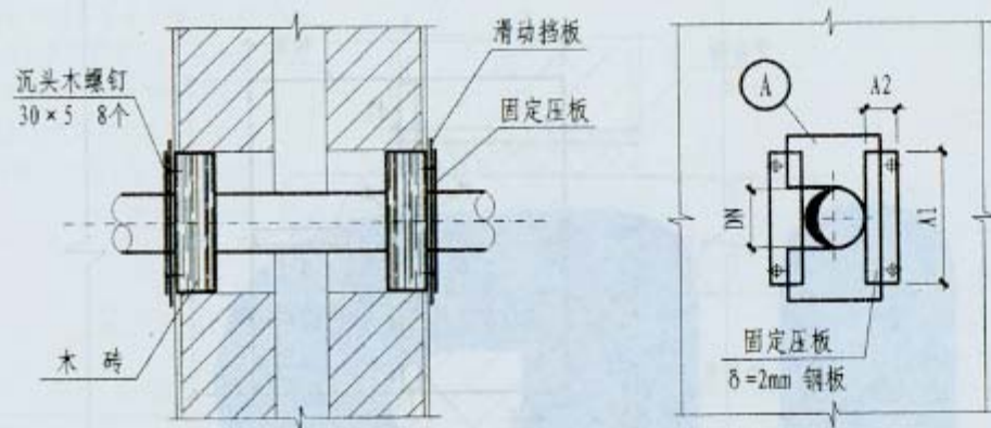
侧面
