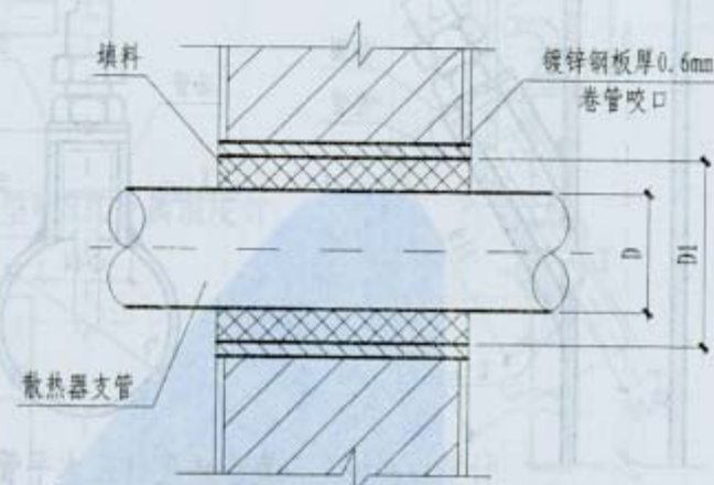
B 型
