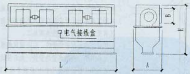
DRKM型立式电热空气幕
