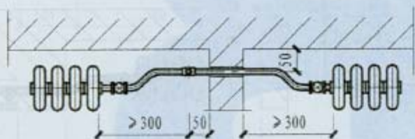
散热器明装平面
