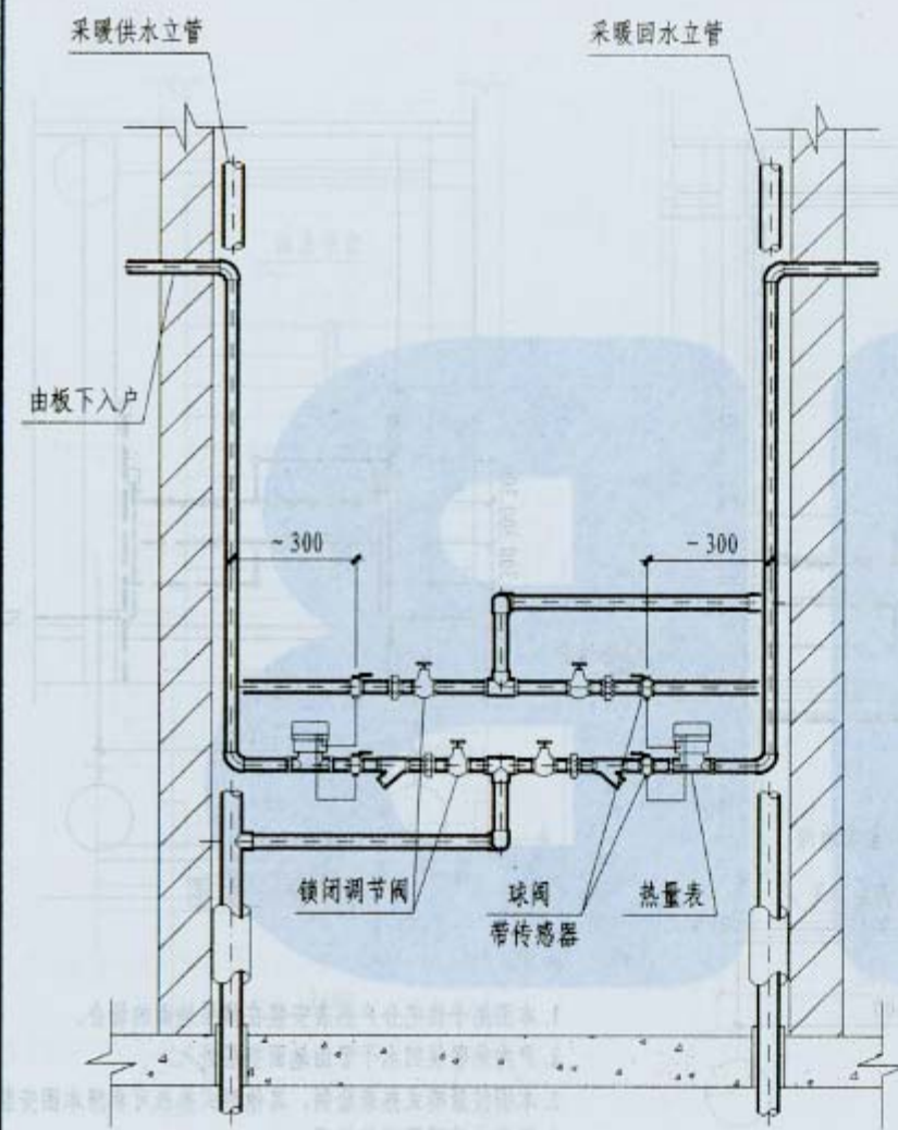
管井剖面图
