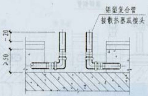
A-A剖面图
