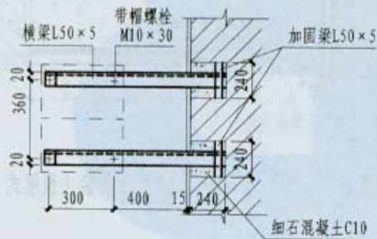
墙上安装
