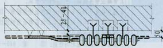
平面图
