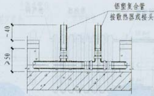
A-A剖面图
