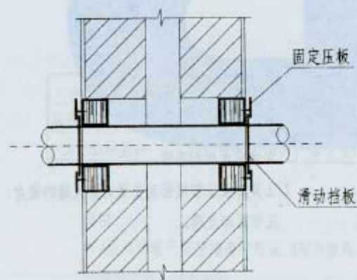
平面
