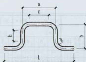
A 型
