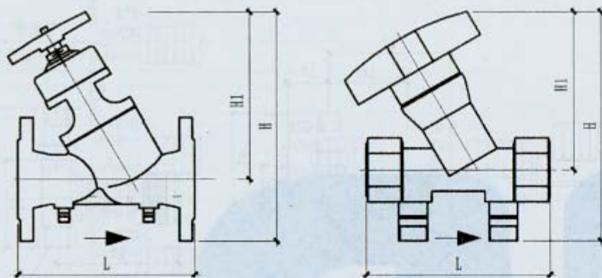
SPF系列数字锁定平衡阀
