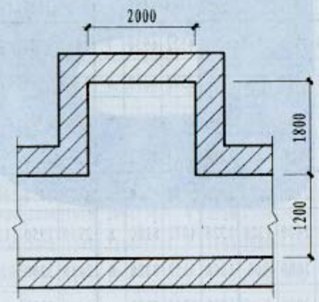
3 号井
