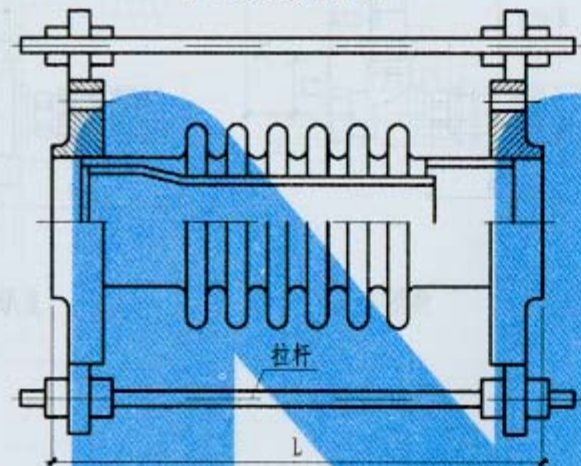
轴向式波纹伸缩节
