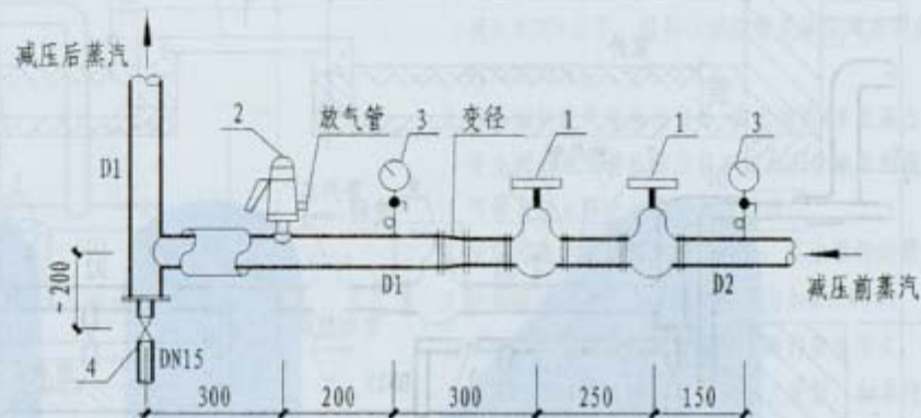
卧式安装
