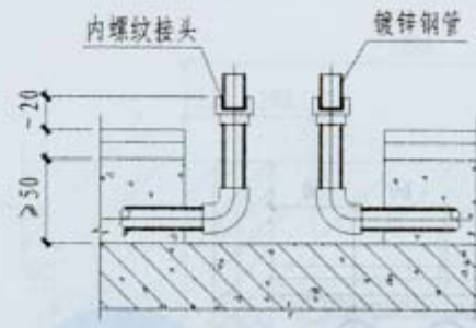
A-A剖图
