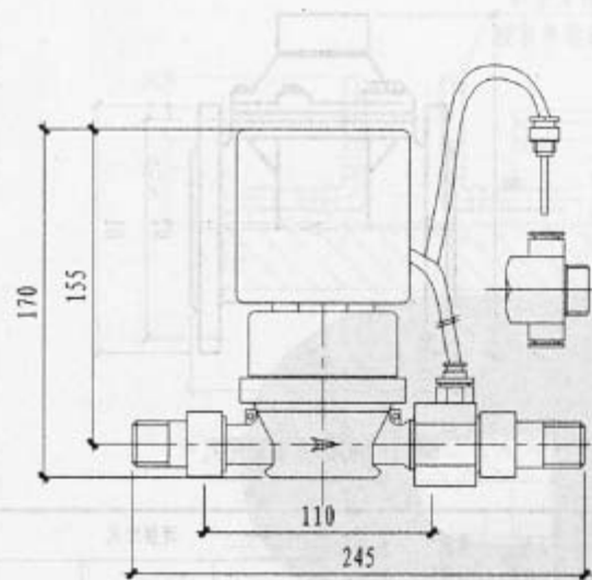
热量表/通讯热量表
