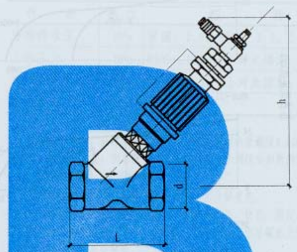
红阀 (mm)
