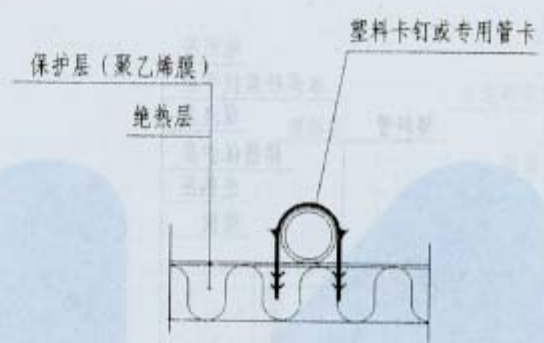
塑料卡钉 (管卡)
