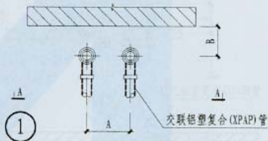
A-A剖面图
