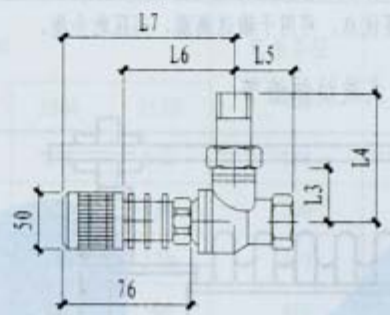
角形
