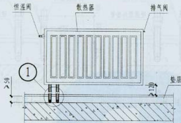
立面图
