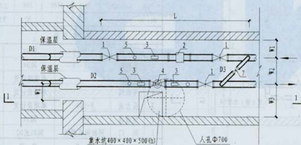
平面图
