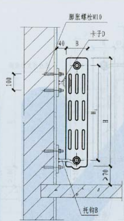
砖墙上挂式安装
