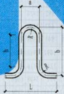
D 型
