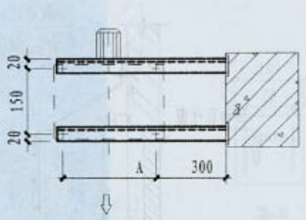
柱上安装 (预埋式)
