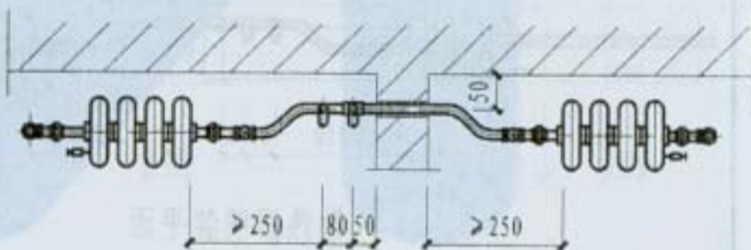
散热器明装平面(用截止阀连接)
