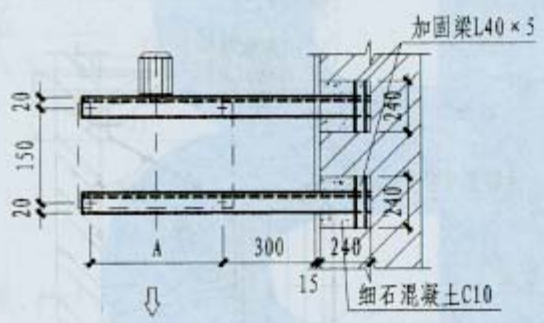
墙上安装
