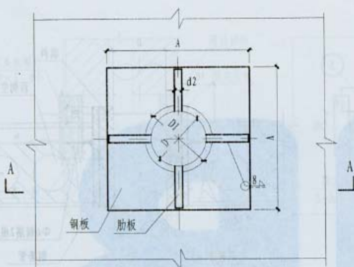
平面
