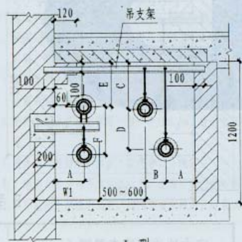
I 型
